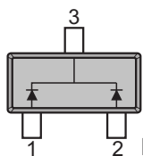
BAT54C
