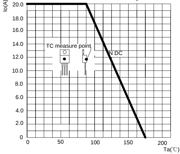
图1: 正向电流降额曲线 FIG1: I_F (AV) \rightarrow T_c Derating
