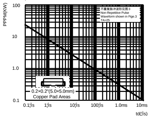
图3：脉冲波形
