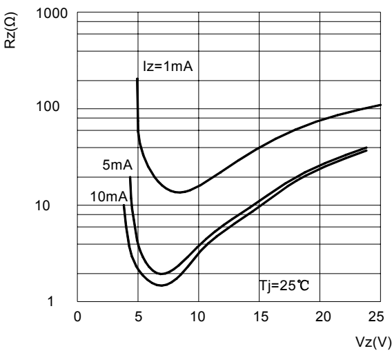
图8：不同齐纳阻抗与齐纳电压的关系 FIG8:Differential Z-Resistance vs. Z-Voltage
