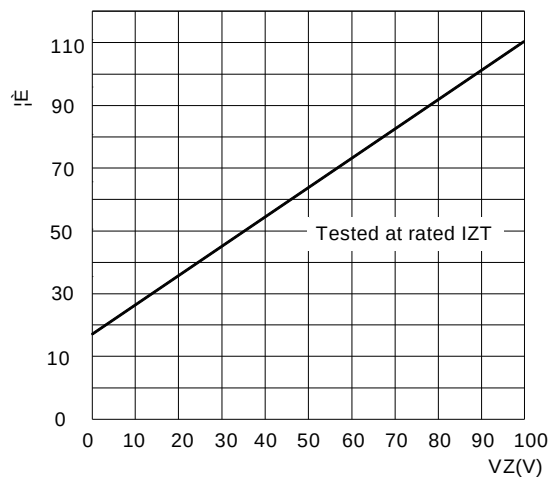
图5：典型反向特性
