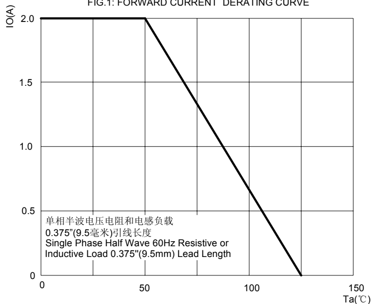
图1: 正向电流降额曲线
